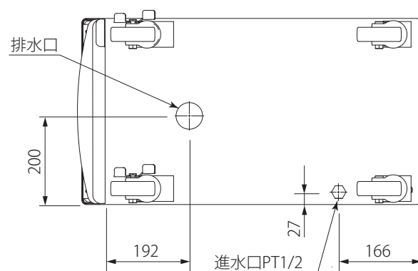
● 底視圖
