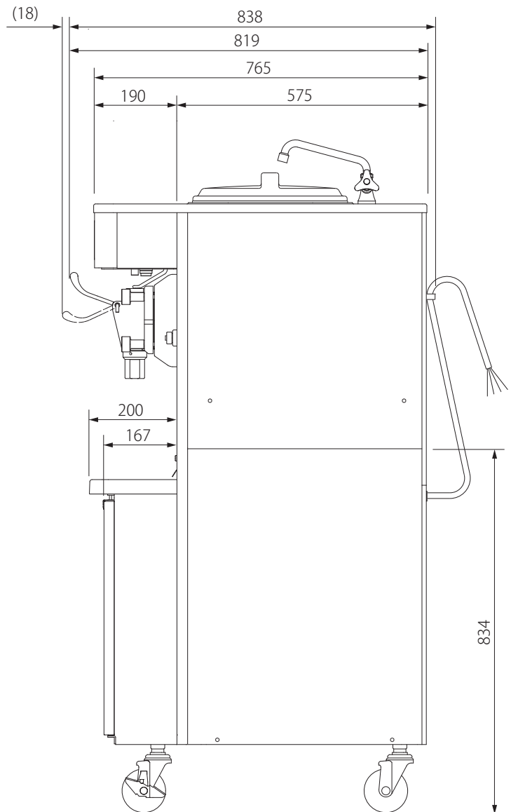
● 側視圖
