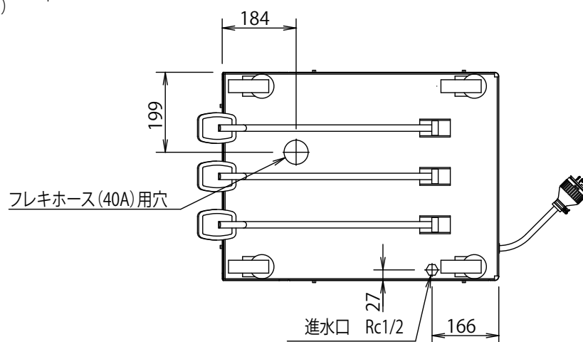
● 底視圖
